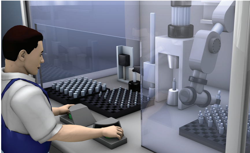
Intégration d'une commande bimanuelle dans le circuit de sécurité via un module d'extension de contacts MSI-CM
